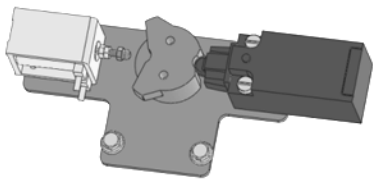
ZURÜCKSETZEN MIT FERNAUSLÖSER
