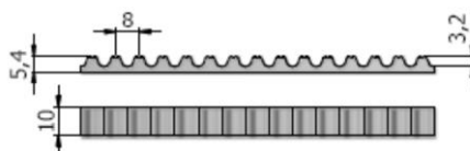
ZAHRAD TYP RPU 8 M10
